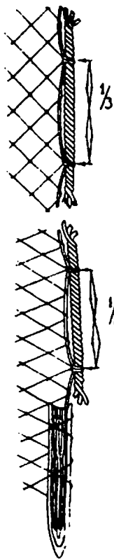
Посадка невода на \frac{1}{3} и на \frac{1}{2}
