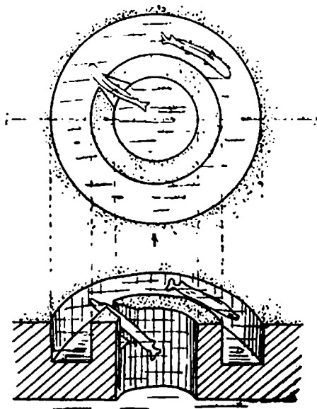
Прорубь с кольцевой канавой. Вид сверху и сбоку (разрез).
